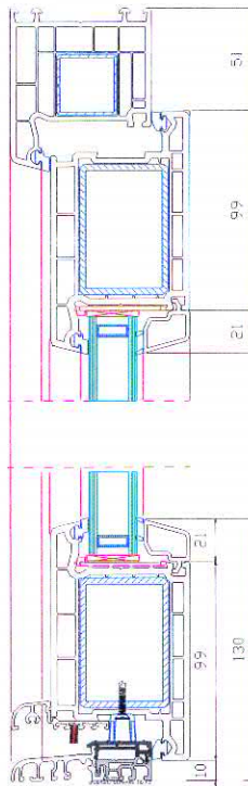
Obrázek 1: Řez rámem VEKA Softline HT 70 – Perfectline - Trendstar
