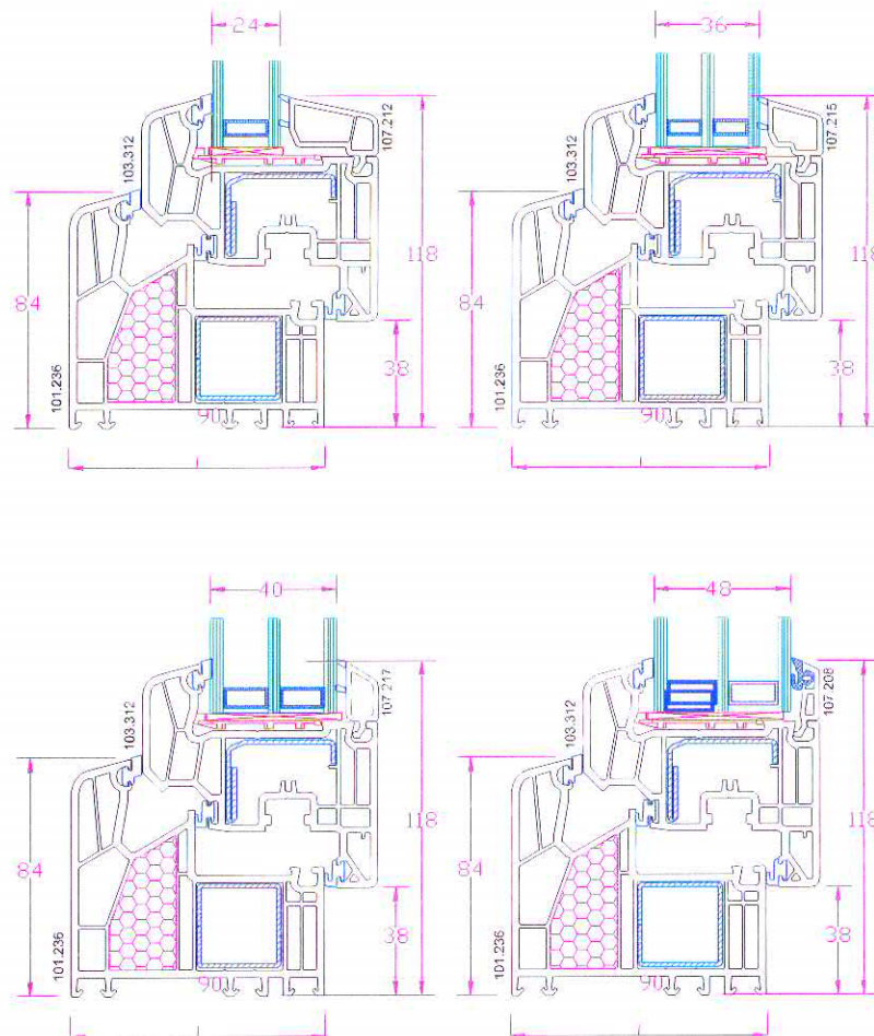
Obrázek 1: Řez rámem VEKA Alphaline 90 MD Climastar
